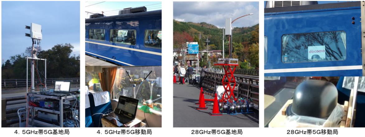
図4. 試験に使用した5G装置
