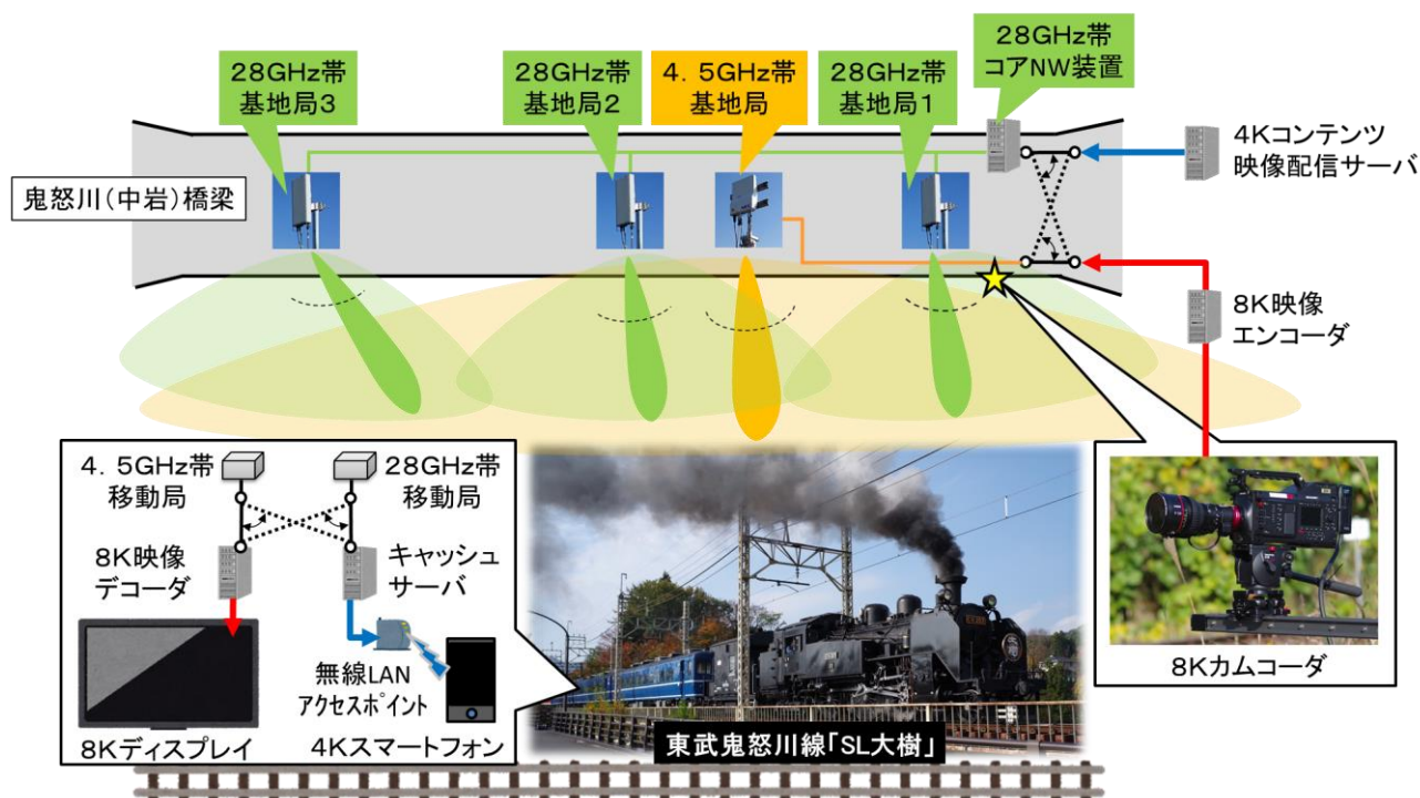
図1. 試験構成
