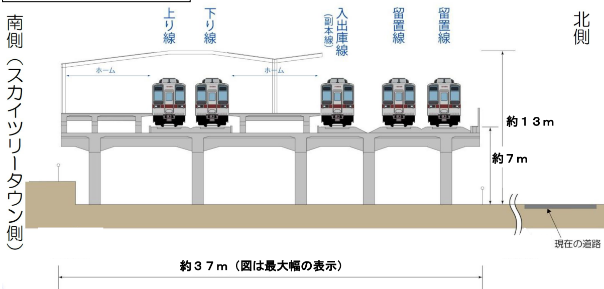
駅部横断面図（イメージ）
