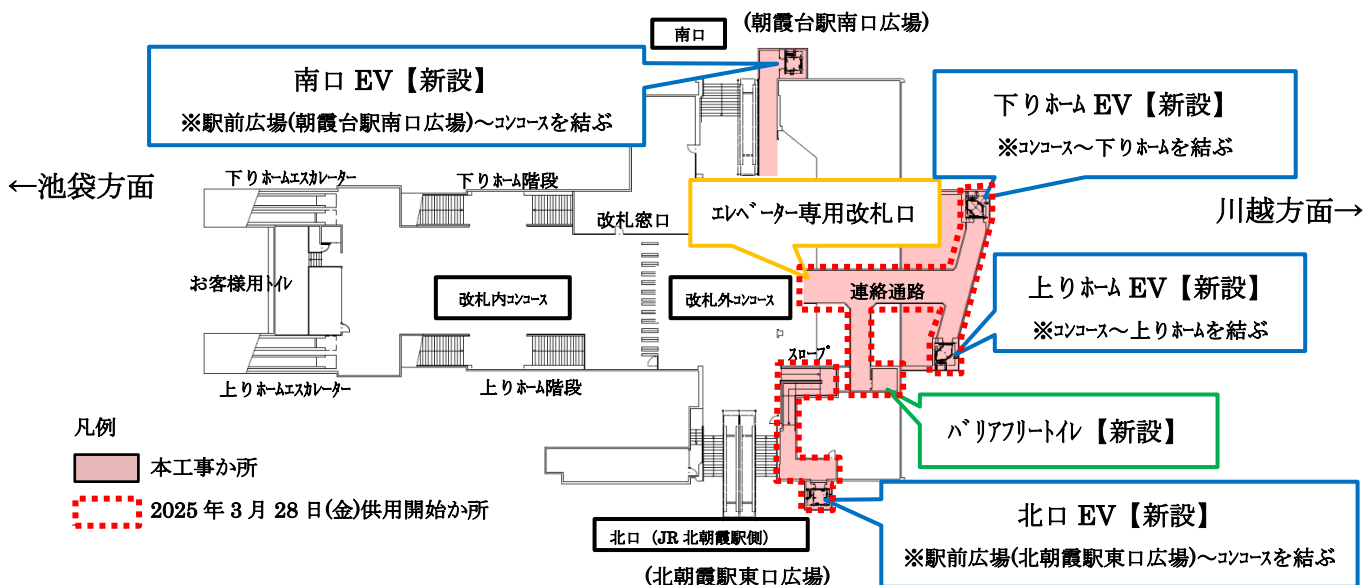
△朝霞台駅 改札階平面図(配置計画)
