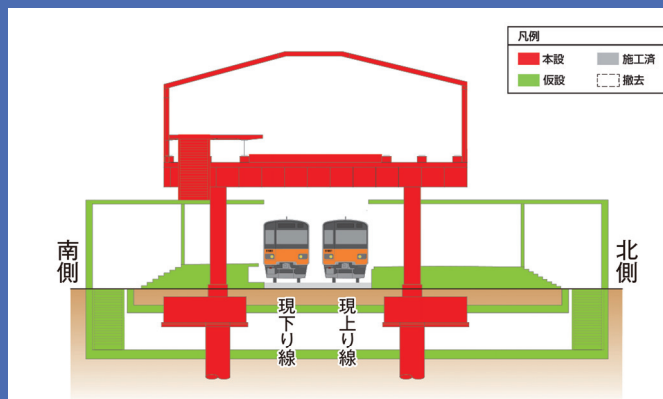
施工順序図(駅部 断面②)
